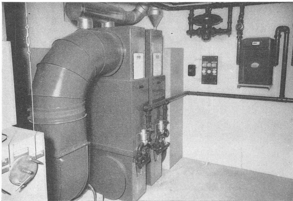
Fig. 3. — Chaufferie du temple de Claren. Générateurs système Strack-Cipag (Arthur Martin, constructeur).
