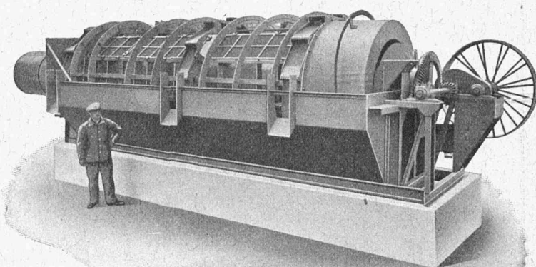
Cribles à oscillations libres. Nouvel appareil de tamisage pour sable et gravier, ainsi que pour toutes applications industrielles.
