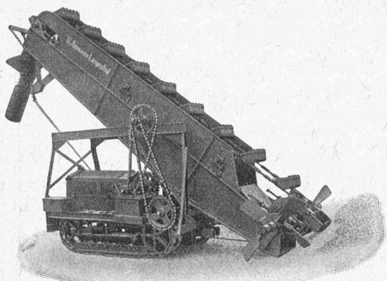
Concasseur moderne complètement en acier et roulements à tonnelets. Robustesse ! Economie ! Rendement élevé !
