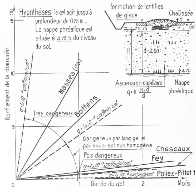
Fig. 10. — Malgré la position exceptionnellement basse, à 4,75 m de profondeur, de la nappe souterraine l'eau parvient encore en grande quantité dans les couches gelées, dans le cas de Bottens et de Mosses 135. Les sols de Fey et de Cheseaux ne deviennent dangereux que par très longs gels. Les autres ne présentent plus aucun danger de formation de lentilles de glace.
