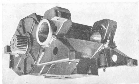
Fig. 7. — Moteur monophasé 240 PS, à carcasse entièrement soudée.
