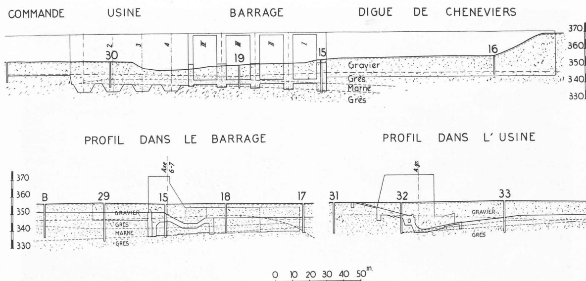
Fig. 6. — Coupes géologiques.
