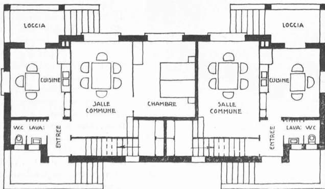
Plan du rez-de-chaussée de l'une des maisons. 1 : 200.
