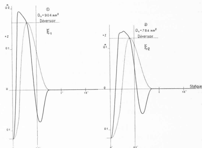
Fig. 6. — Chambre d'équilibre différentielle à amortissement immédiat. Fermetures progressives linéaires de 7 à 0 dm 3 /s. Rapidité de manœuvre de l'obturateur \xi_1 = 0,778 \text{ dm}^3/\text{s}^2 \xi_2 = 0,394 \text{ dm}^3/\text{s}^2 . Galerie d'amenée de 70,84 m de longueur et de 150 mm de diamètre. Les sections respectives du tube et du réservoir sont de 403 et 1116 cm 2 .
