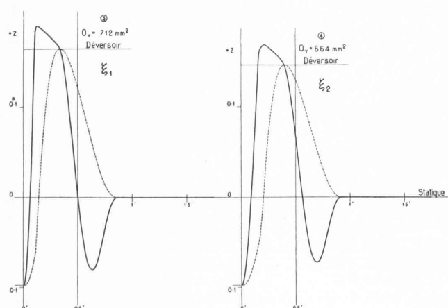
Fig. 5. — Chambre d'équilibre différentielle à amortissement immédiat. Fermetures progressives linéaires de 5 à 0 dm 3 /s. Rapidité de manœuvre de l'obturateur \xi_1 = \frac{dQ}{dt} = 0,778 \text{ dm}^3/\text{s}^2 \xi_2 = \frac{dQ}{dt} = 0,394 \text{ dm}^3/\text{s}^2 . Galerie d'amenée de 101,74 m de longueur et de 150 mm de diamètre. Les sections respectives du tube et du réservoir sont de 403 et 1116 cm 2 . Les chiffres entourés d'un cercle renvoient aux numéros des essais figurant sur le tableau numérique.
