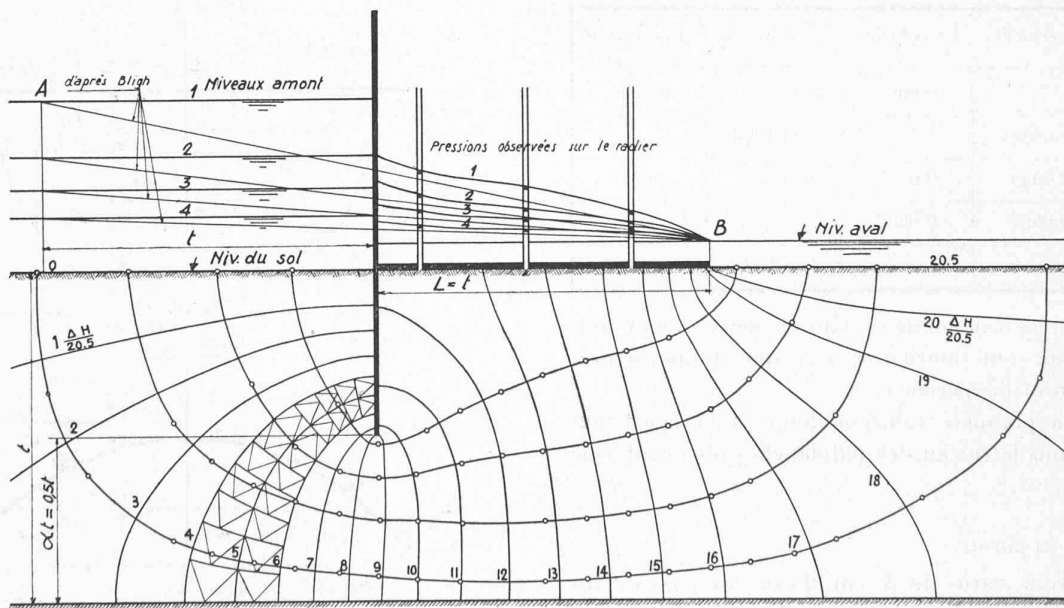
Fig. 11. — Ecoulement sous un rideau de palplanches avec radier aval de longueur égale à l . Lignes de courant observées en laboratoire.
