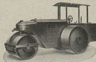
Rouleau-compresseur trijante
