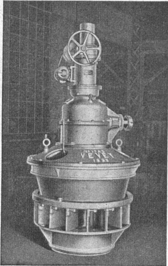
Turbine Kaplan 40 CV.
