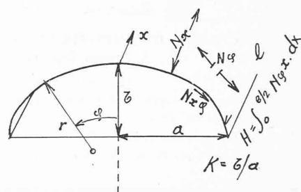
Fig. 3. — Voûte elliptique.
