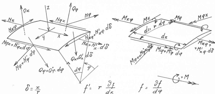
Fig. 5. — Efforts élémentaires dans la voûte fléchie.
