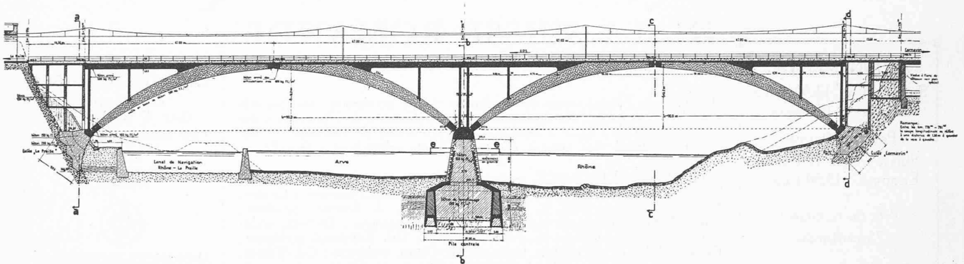
Coupe longitudinale dans l'axe de la voie.
