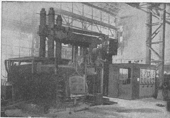
Four triphasé à acier de 15 tonnes, équipé de régulateurs automatiques ultra-rapides, système Sécheron.
