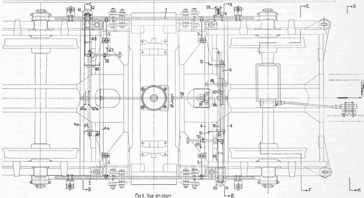
Fig. 10, Elévation
