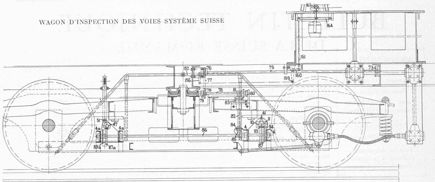
Fig. 9, Coupe longitudinale
