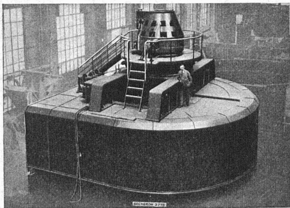
Alternateur de 27 500 KVA, 18 880 V, 136 t/m pour l'Usine du Verbois sur le Rhône. Montage pour essais en atelier.
