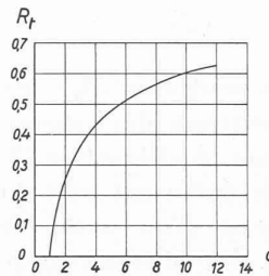
Fig. 2. — Dépendance entre le rendement thermique R_t et le taux de compression c pour le cycle a), sans récupération.
