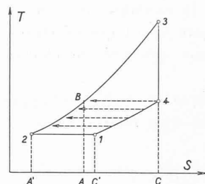
Fig. 7. — Diagramme T—S du cycle b ), avec récupération.
