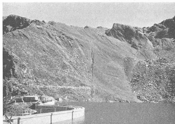
Fig. 5. — L'Illsee.
