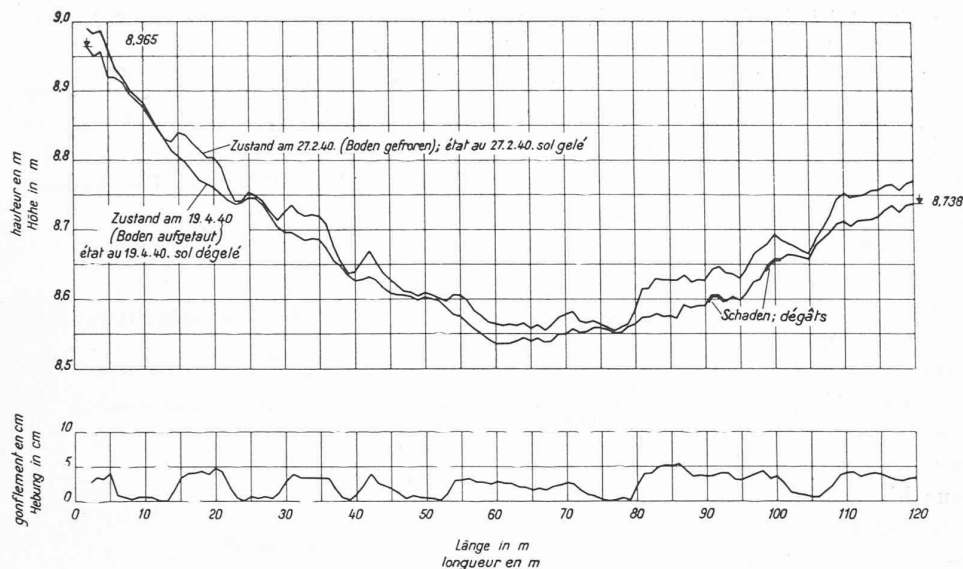
Fig. 44. — Observation des effets du gel à Ebikon. Gonflements mesurés suivant le profil en long.
