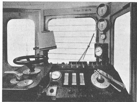
Fig. 27. — Autorail, cabine de mécanicien.
