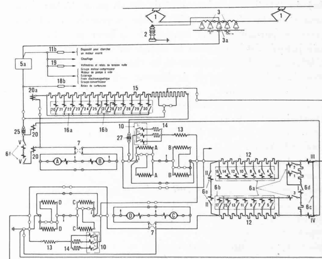
Fig. 19. — Schéma simplifié des circuits de traction, de récupération et de freinage rhéostatique.
