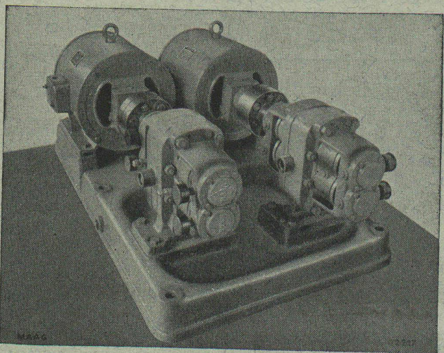
Groupe de deux pompes pour refolement d'eau de savon à 40 atm.
