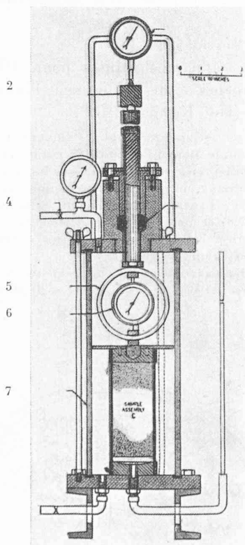
Fig. 3. — Schéma d'un appareil triaxial.
