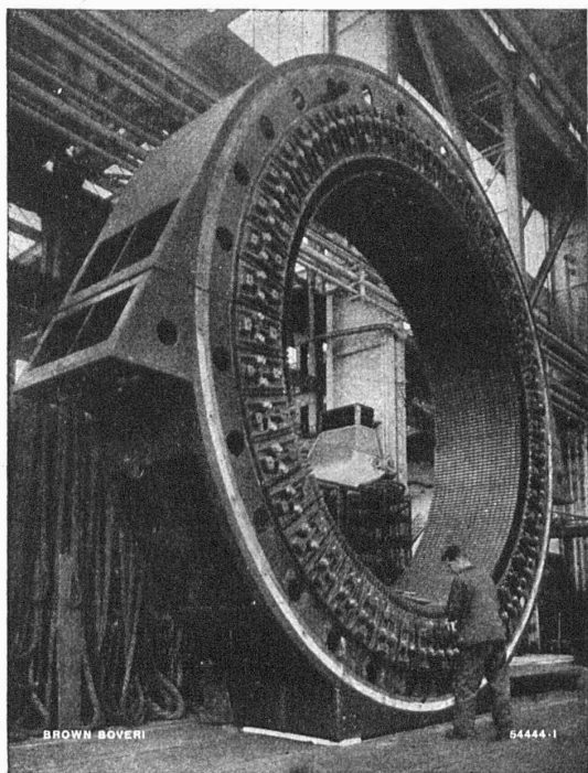
Travaux d'usinage du stator d'un alternateur de grande puissance.
