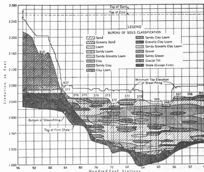
Fig. 13. — Barrage de Fort Peck, Coupe géologique schématique suivant l'axe longitudinal du barrage rive droite (zone de glissement).
