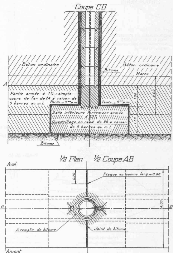
Fig. 34. — Détail d'un joint selon le projet initial.
