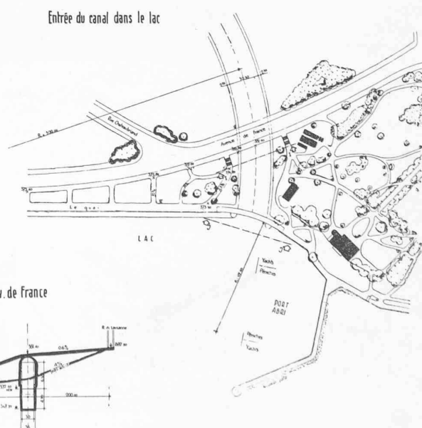
Plan de l'entrée du canal dans le lac. — Echelle 1 : 5000.
