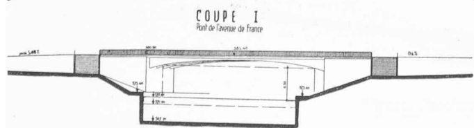
Coupes du canal. — Echelle 1 : 1000.
