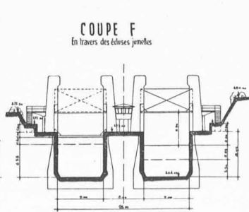
Coupes — Echelle 1 : 1000.
