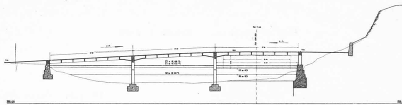
Pont de Soutierre. — Echelle 1 : 1600.
