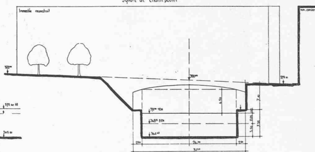
COUPE C Square de Chantepoulet
