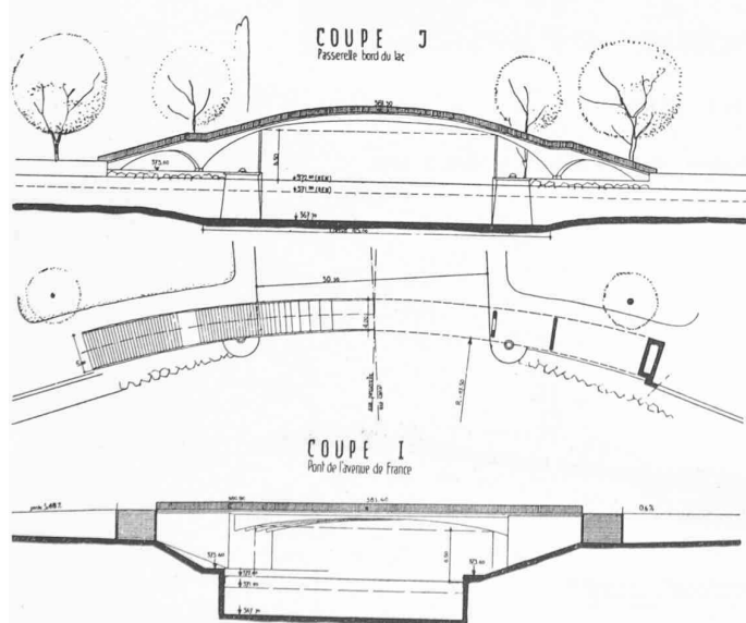
Coupes du canal. — Echelle 1 : 1000.
