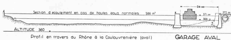
Profil en travers du Rhône à la Coulouvrenière (aval)
