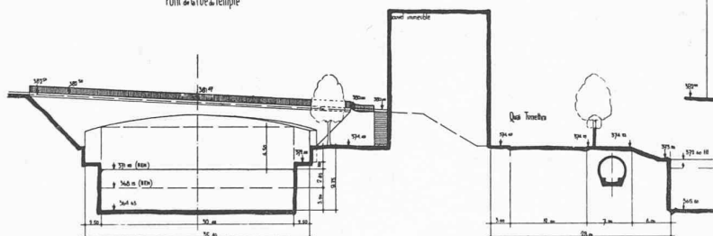
COUPE B Pont de la rue du Temple
