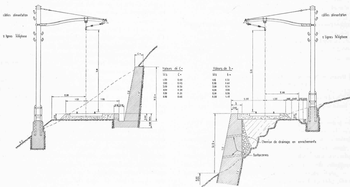
Fig. 10. — Profils en travers types du Chemin de fer Montreux-Oberland bernois.
