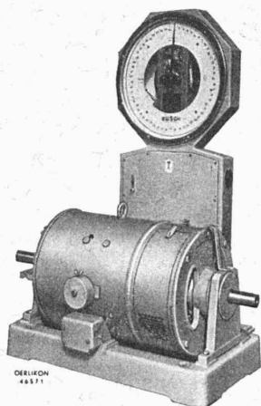
Dynamomètre moderne type 57, avec balance rapide de précision. Puissances : comme génératrice : 3...45 kW comme moteur : 3,5...55 kW Vitesses : 400...4000 t/min
