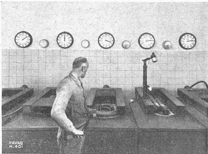
Vue partielle d'une installation de compteur de durée à signaux, pour un atelier de trempe. Le tableau de commande permet de régler à l'avance la durée d'opération prévue, avec signalisation acoustique ou lumineuse de fin d'exécution. Retour à zéro ou répétition automatique des signaux.
