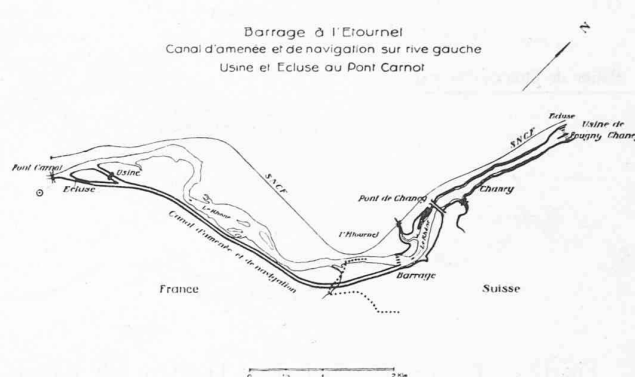
Fig. 10. — Palier de l'Etournel. Solution 4 d'aménagement : barrage sur le Rhône établi à environ 800 m en amont de l'extrême frontière ; canal d'amenée d'eau à l'usine et de navigation, long d'environ 4,5 km, placé sur la rive gauche ; usine hydro-électrique et écluse de navigation placés légèrement en amont du Pont Carnot.
