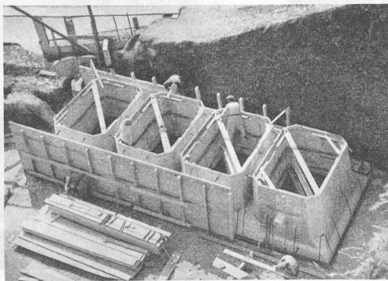
Fig. 6. — Coffrages de la caisse de havage sur la rive droite.
