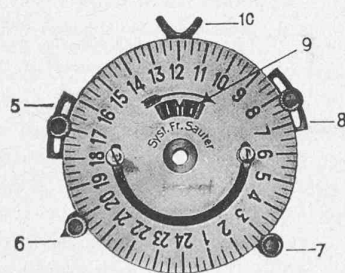
Fig. 15. — Cadran à correction astronomique.
