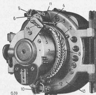
Fig. 16. — Cadran à correction astronomique.
