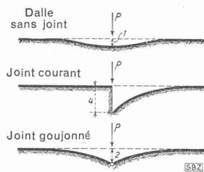
Fig. 36. — Affaissement d'un revêtement sous l'effet d'un essieu isolé.
