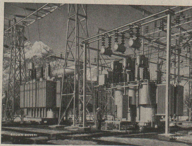
Poste de transformation récent d'une centrale suisse. Le refroidissement des transformateurs est assuré par des radiateurs à tubes et le réglage de la tension se fait par des commutateurs de prises, à commande par ressort, montés directement sur les transformateurs.
