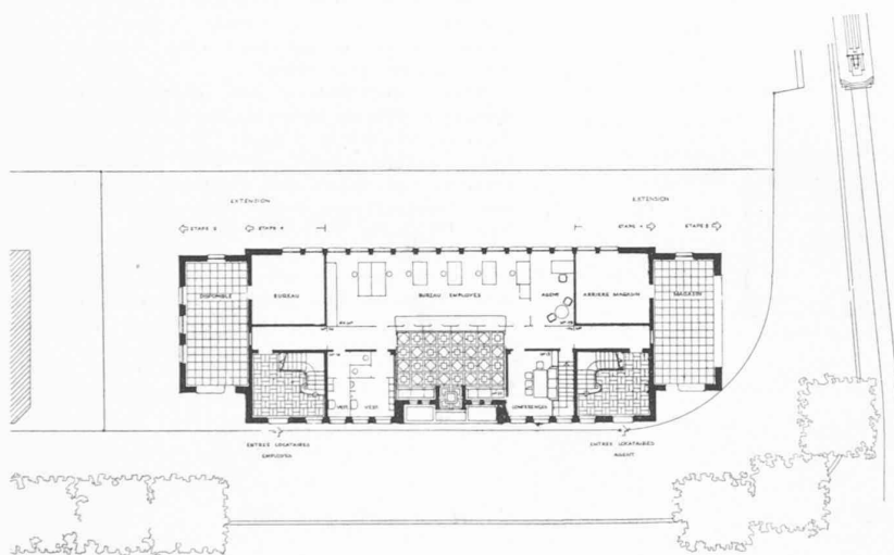
Rez-de-chaussée. — Echelle 1 : 500.
