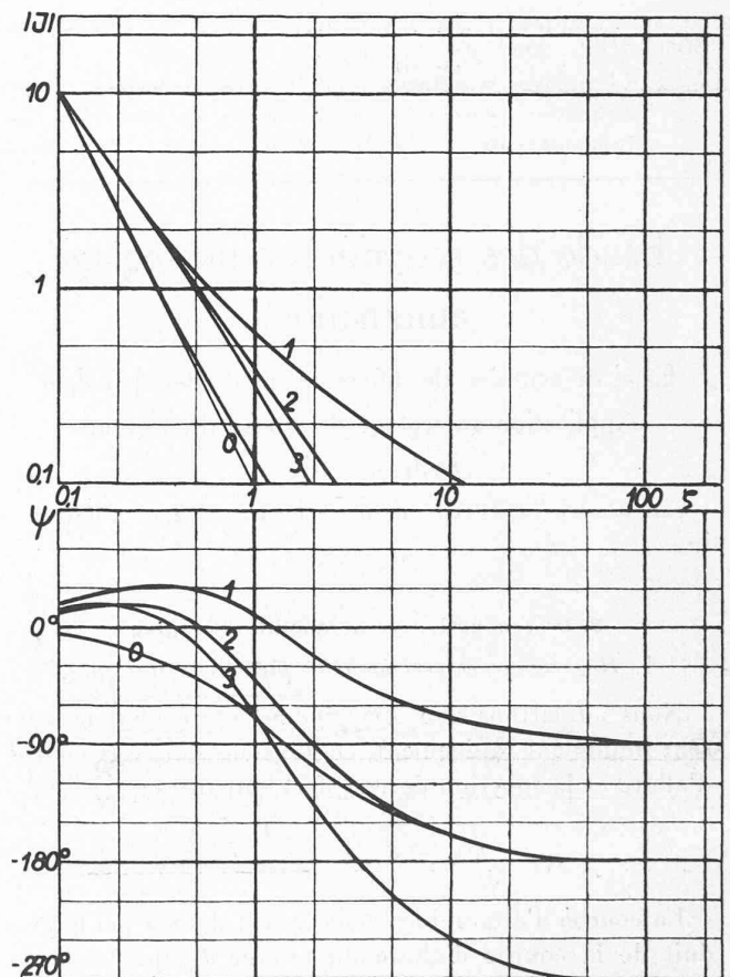
Fig. 42. — Courbe d'allure du réglage ouvert sous forme cartésienne avec régulateur accéléro-tachymétrique à vitesse limitée.
