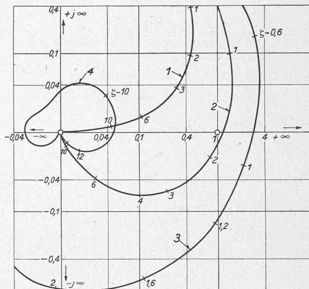
Fig. 16. — Représentation vectorielle de la courbe d'allure du réglage.
