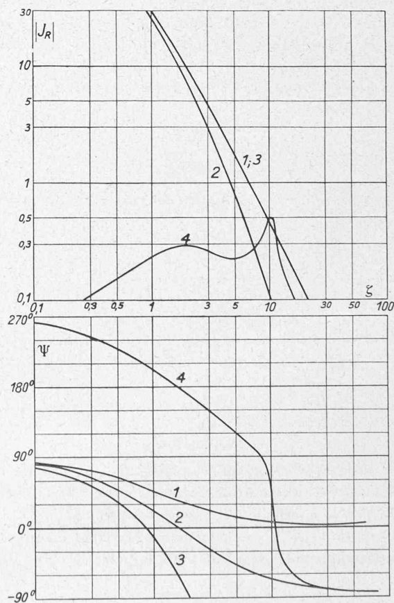
Fig. 17. — Représentation cartésienne de la courbe d'allure du réglage.
