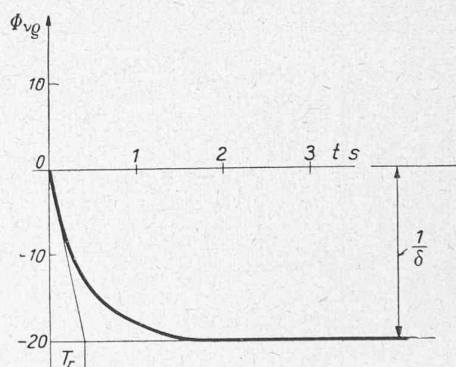
Fig. 9. — Courbe de réponse du régulateur statique.
