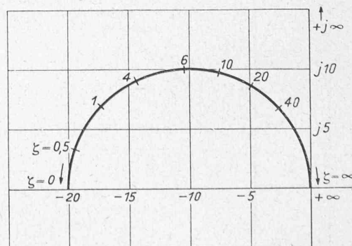
Fig. 10. — Courbe d'allure du régulateur statique.
