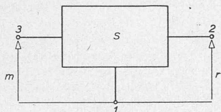
Fig. 2. — Représentation schématique d'un servomoteur sous la forme d'un tripôle.
