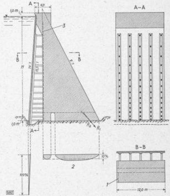
Fig. 3. — Barrage avec écran amont étanche.
