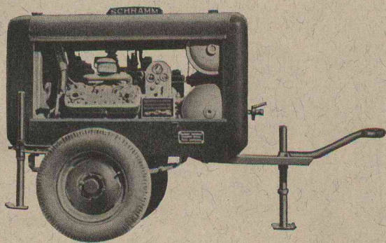
Type 60 de 1,7 m 3 asp. effective par minute
