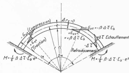
Effet d'un état de température variant linéairement de -\Delta\tau sur l'intrados à +\Delta\tau sur l'extrados
