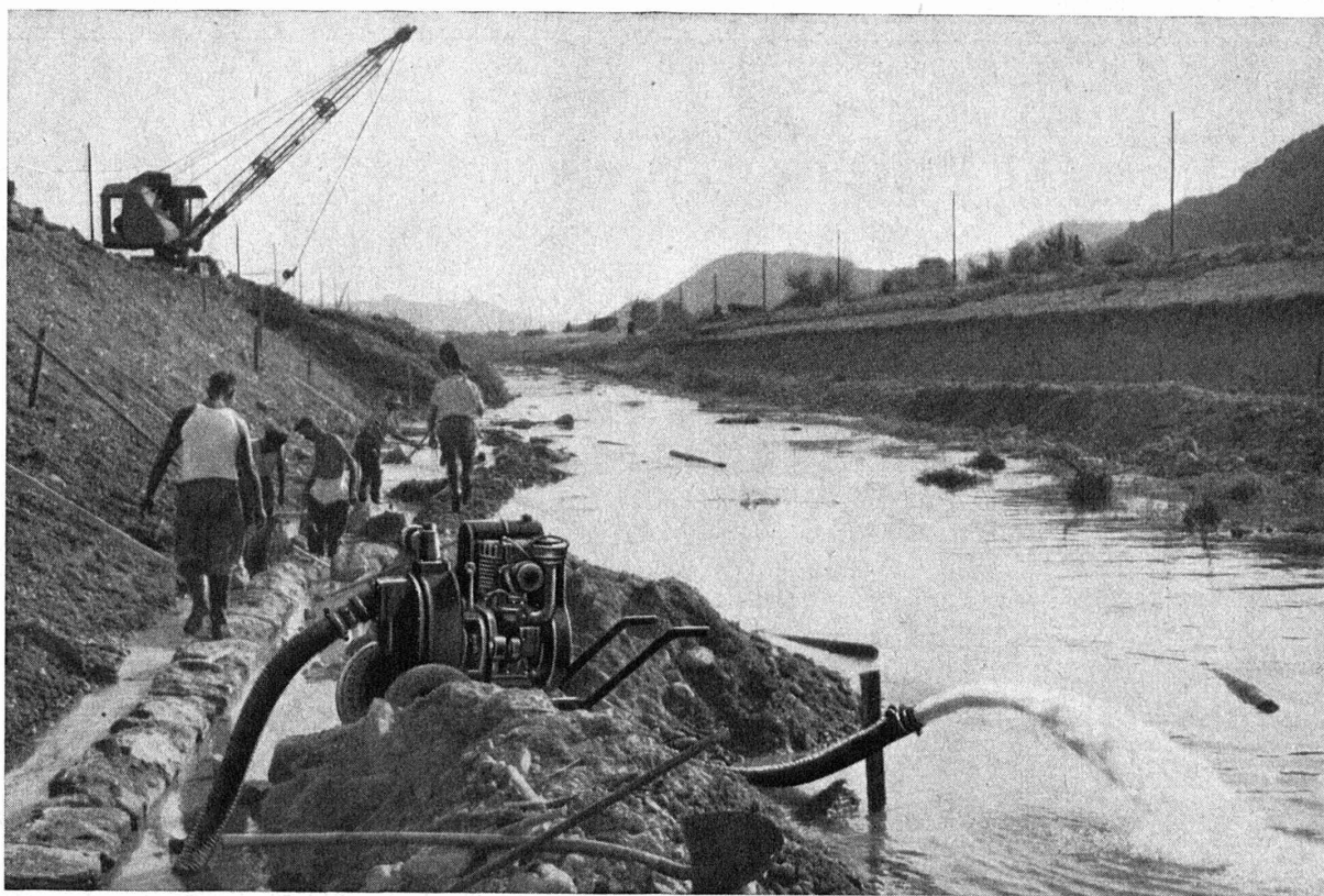
Pompe centrifuge auto-aspirante MARLOW en action.
