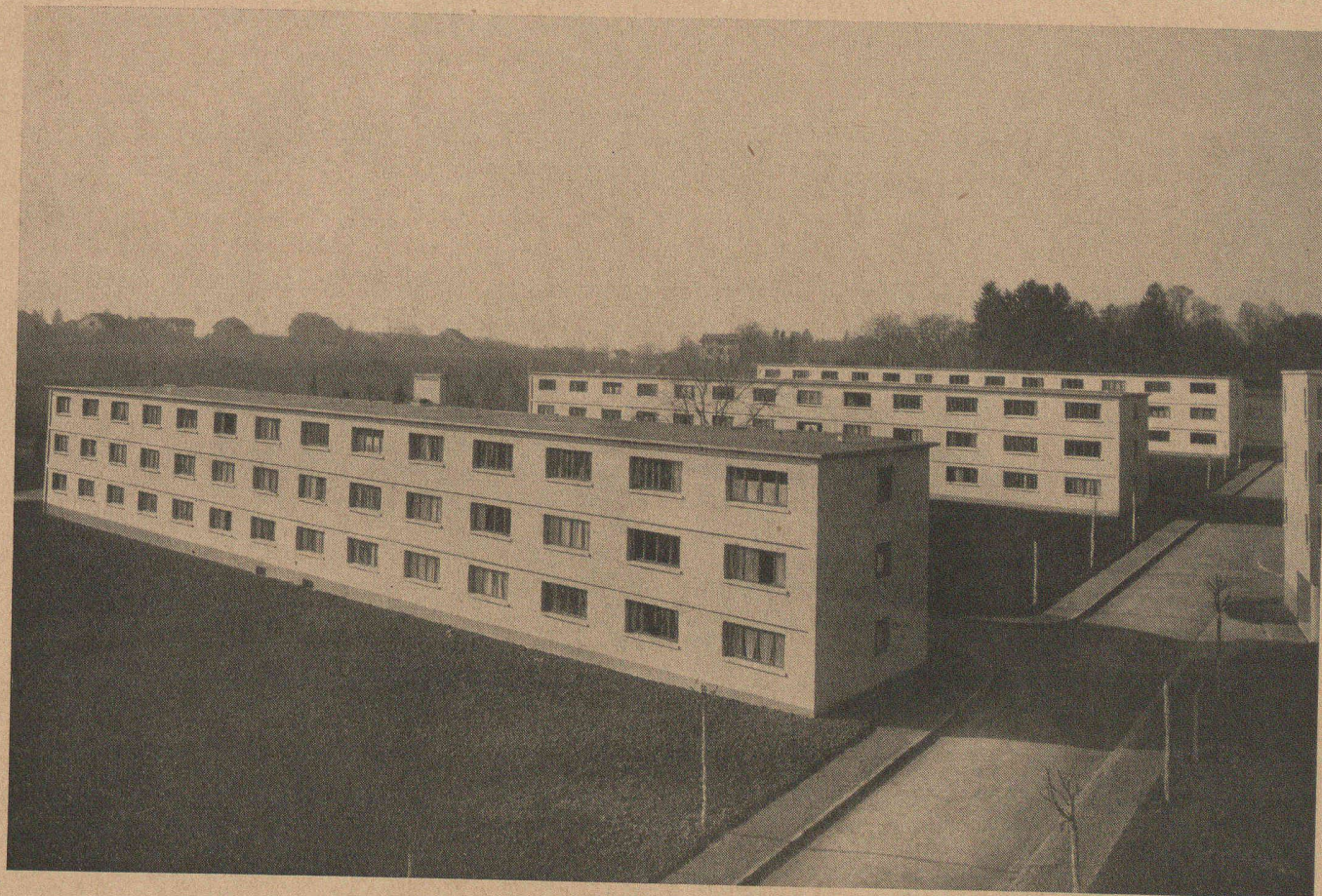
Cité Vieusseux, Genève. — Étanchéité des toitures-terrasses exécutées en asphalte souple « Système Hirschy » il y a vingt ans
