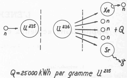
Fig. 3. — Représentation schématique du processus de fission de l'uranium.
