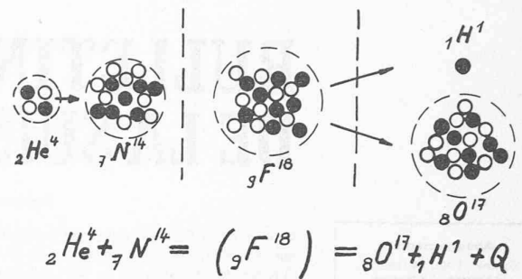
Fig. 2. — Exemple de réaction nucléaire. Un noyau d'hélium (particule \alpha ) accéléré entre en collision avec un atome d'azote. Le noyau intermédiaire formé (fluor) est très fortement excité et, après une durée de vie négligeable, expulse un noyau d'hydrogène (proton) et donne naissance à un noyau d'oxygène de masse 17.
