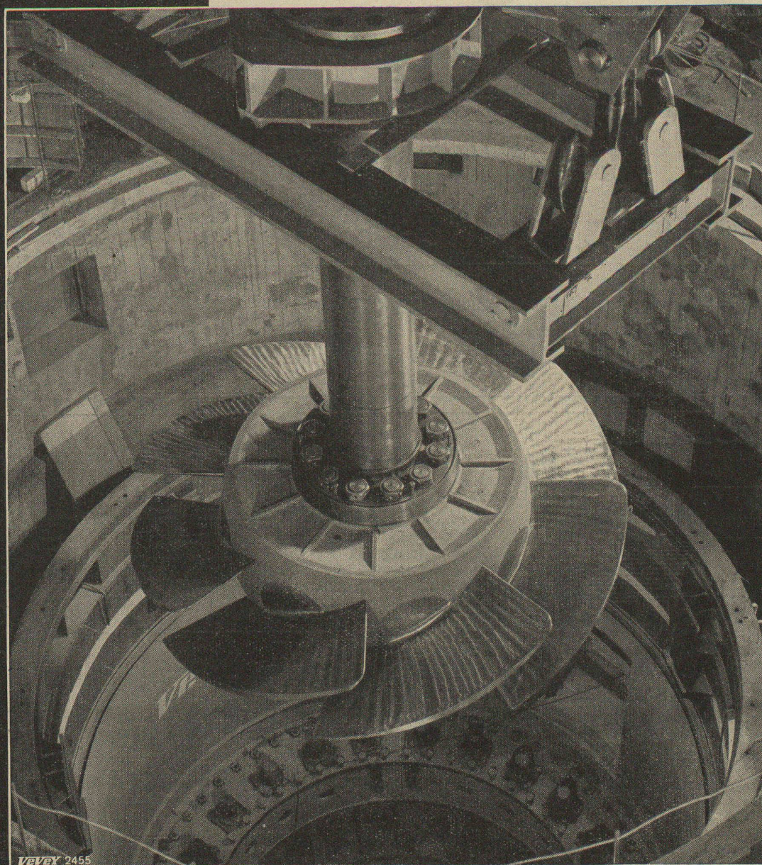
Usine de Lavey, roue Kaplan de 33 650 ch
