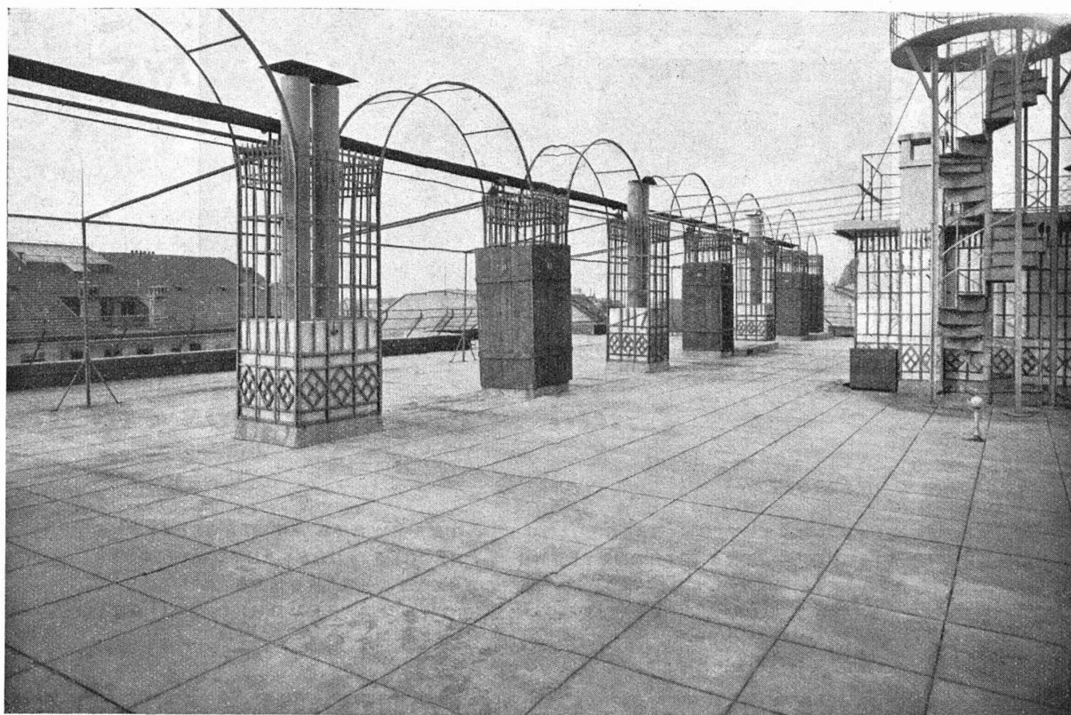
Hôtel de la Résidence, Genève. — Etanchéité des toitures-terrasses, exécutées il y a 22 ans, en asphalte souple « Système Hirschy ».
