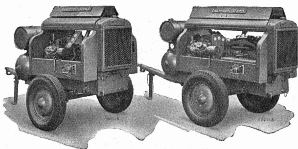
modèle D-60 modèle D-85 transportables, avec moteur à benzine
