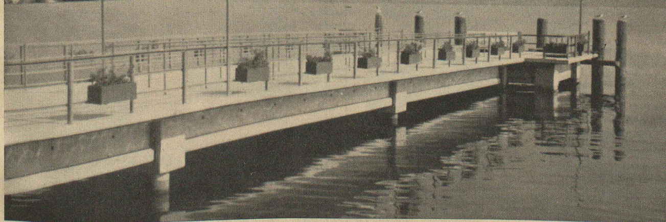
Débarcadère de Nyon reconstruit en 1947 en béton précontraint — Exécutant : ENTREPRISE LOSINGER & Cie S. A., Lausanne A gauche en haut : Deux ancrages de câbles et le vérin de précontrainte (voir page 12 du présent numéro).
