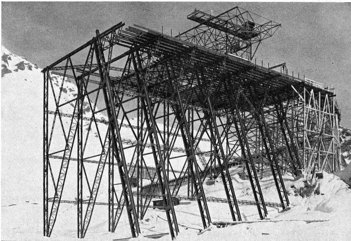
Estacade des blondins du barrage de Salanfe, exécutée par les Ateliers de Constructions Mécaniques de Vevey S. A.
