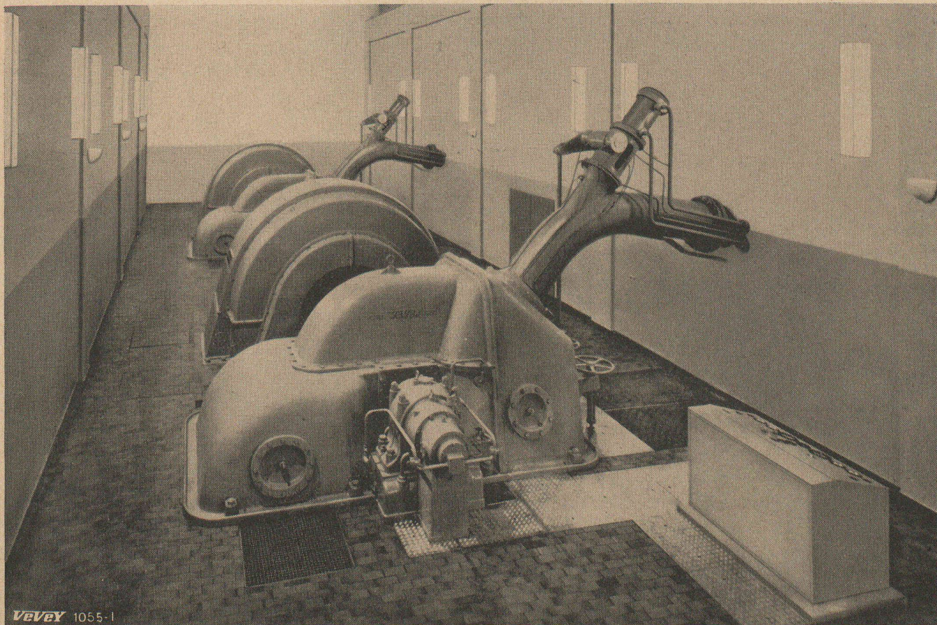
Vue de la salle des machines de la Centrale de Sasselto des Forces motrices de la Calancasca S. A. Les deux turbines de 14 130 ch chacune ont été livrées, avec leurs régulateurs, par les Ateliers de Constructions Mécaniques de Vevey S. A.
