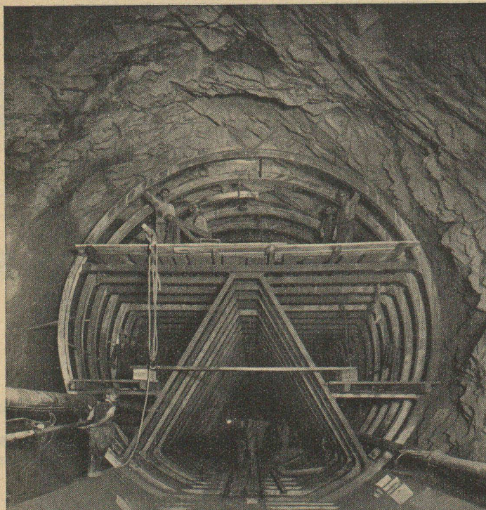
Tunnel d'amenée de l'Usine de Lavay exécuté en consortium Conduite du chantier du lot 2:
