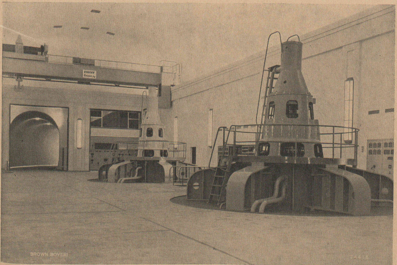
Salle des machines de l'usine souterraine de Lavey, de la ville de Lausanne, avec deux alternateurs à axe vertical Brown Boveri de 29 400 kVA chacun, 10 000 V, 50 Hz, 214 t/min.
